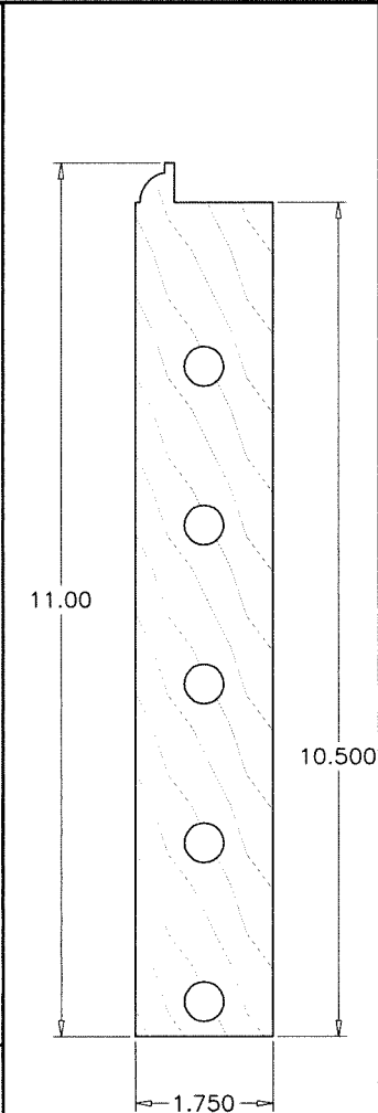
⑥ DOOR SIDE RAIL
